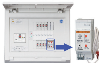
▲分電盤タイプ
